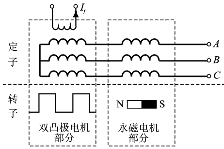
图10 并列式混合励磁电机示意图
