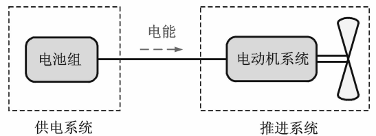
图4 纯电动电推进基本架构
