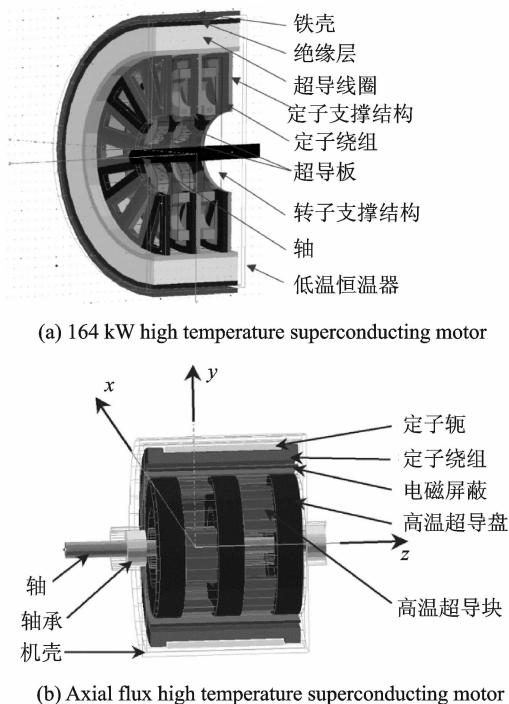
图 14 高温超导电动机
