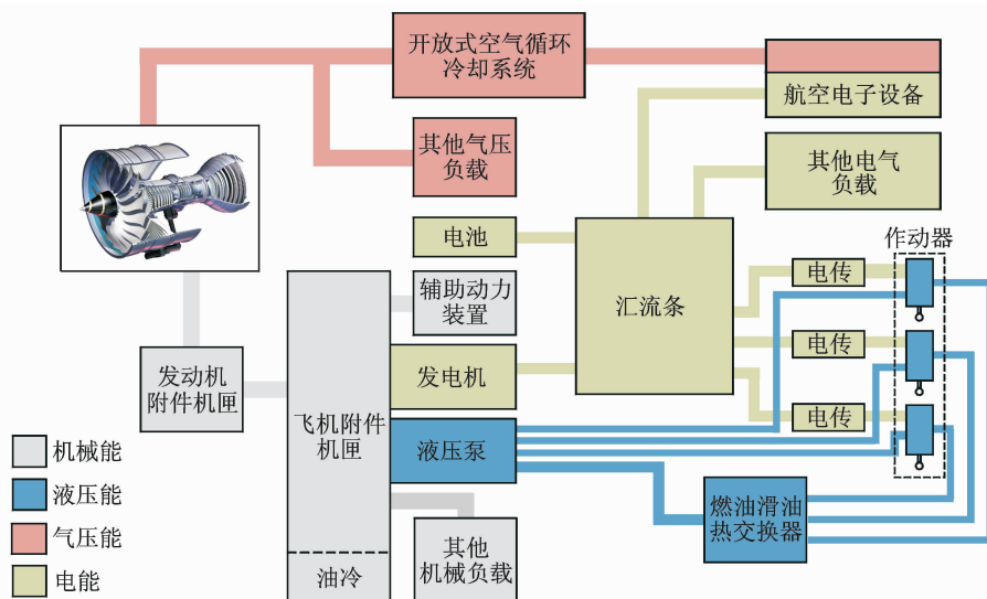
图 1 传统飞机二次能源结构
