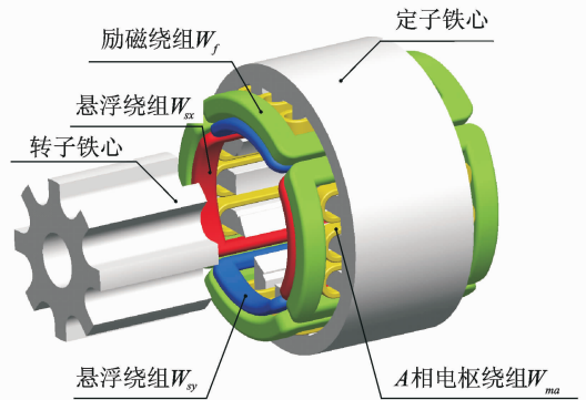
图 12 无轴承电励磁双凸极电机
