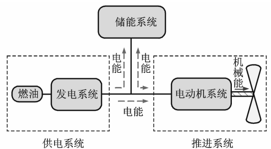
图5 混合电推进基本架构
