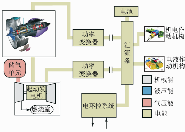
图2 全电飞机二次能源结构
