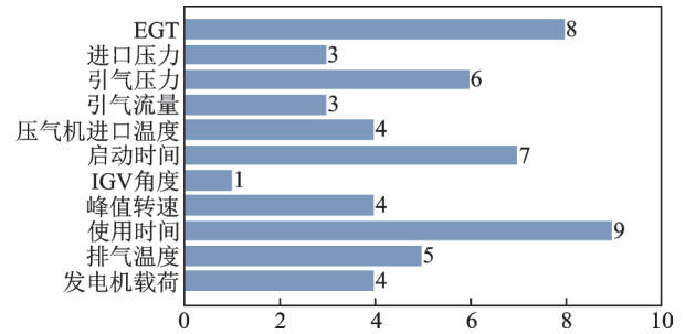
图3 递归特征消除得分情况
