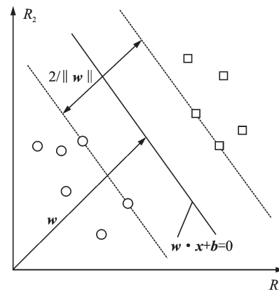
图 2 最优超平面
