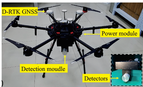
图 1 无人旋翼机机载放射性监测系统
