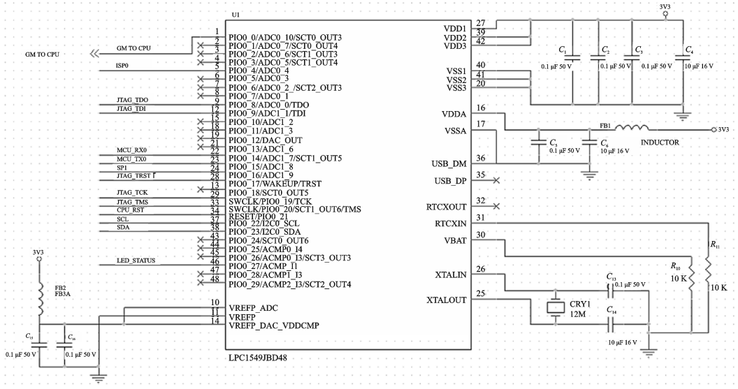
图3 LPC 芯片功能引脚分配设计
