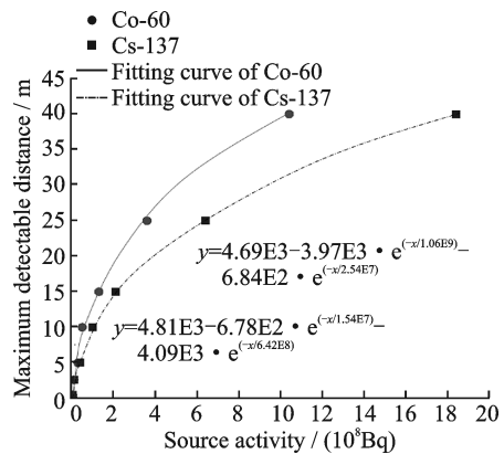
图 8 源活度-最大可探测距离关系曲线
