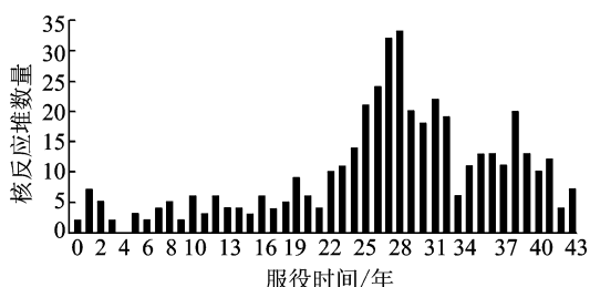
图3 全世界正在运行核动力反应堆(核电站)服役时间分布图 [2]
